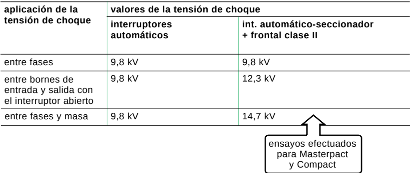
Fig. 12: Prueba de rigidez a las ondas de choque para los interruptores industriales. Durante los diversos ensayos, no debe de producirse ninguna descarga entre fases, entre contactos abiertos o entre fase y masa.
